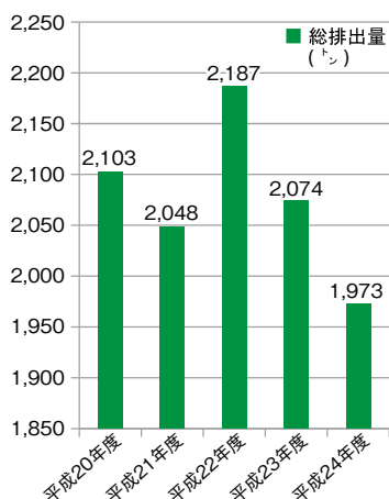
温室効果ガス総排出量の推移
