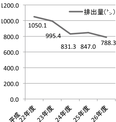
平成26年度役場など町関連施設の温室効果ガス排出量の推移
