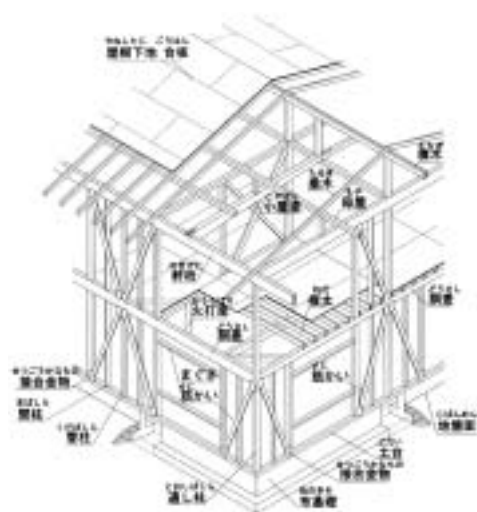
在来軸組構法の構造図
